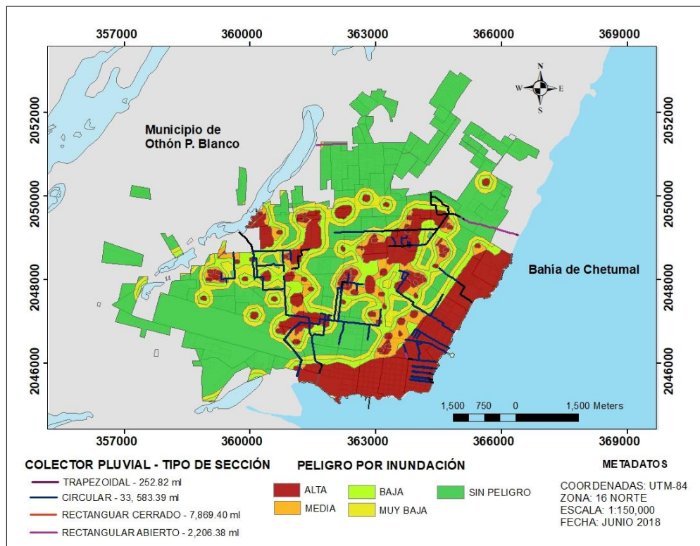
Figura 5.4. Sistema de drenaje pluvial
